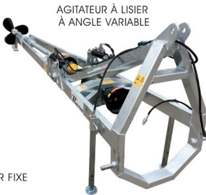
Agitateur à lisier à angle variable
